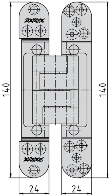
PIVOTA® DX 38 3-D CP „Design“
