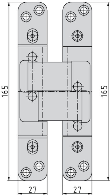
PIVOTA® DX 35 2-D „LT“
